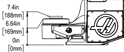
A5 PLATTER
